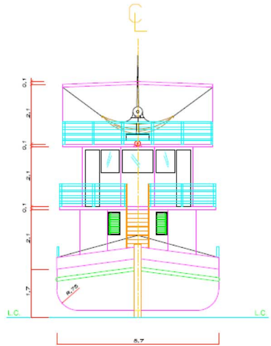
VISTA PROA ESC: 1/50
