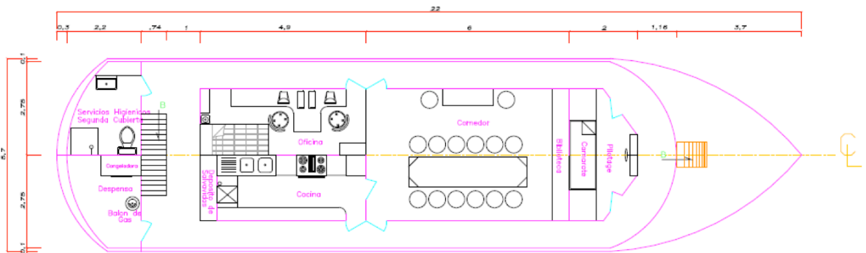
SEGUNDA CUBIERTA ESC: 1/50
