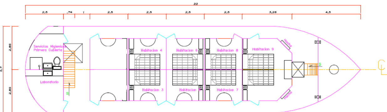
PRIMERA CUBIERTA ESC: 1/50
