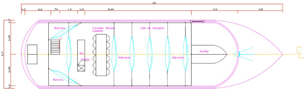
TERRAZA ESC: 1/50
