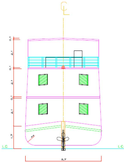
VISTA POPA ESC: 1/50
